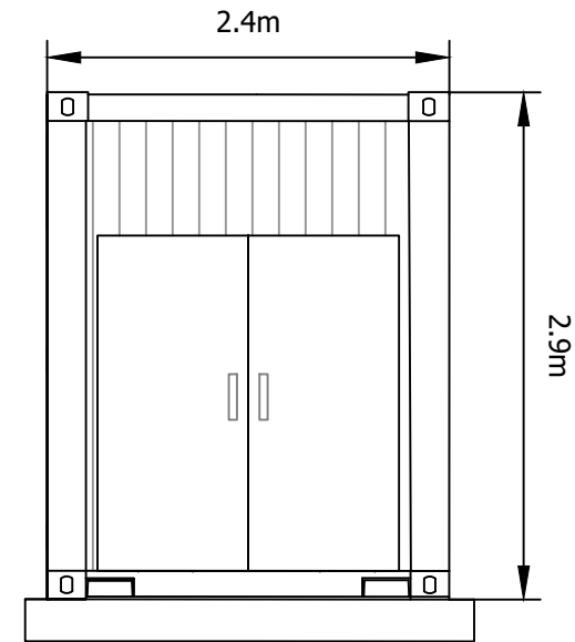
END ELEVATION
